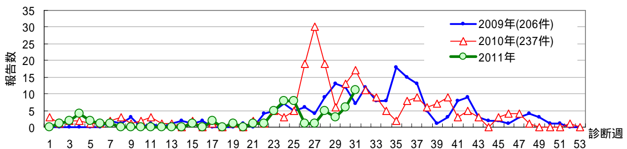
図3 腸管出血性大腸菌感染症診断週別発生状況 (愛知県、無症状病原体保有者含む、2009年1週~2011年31週、8月10日現在)
